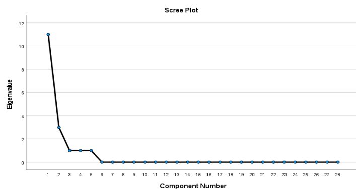
شکل ۲- نمودار سنگریزه
