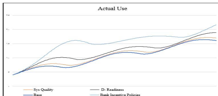
شکل ۱۷. مقایسه سناریوها
