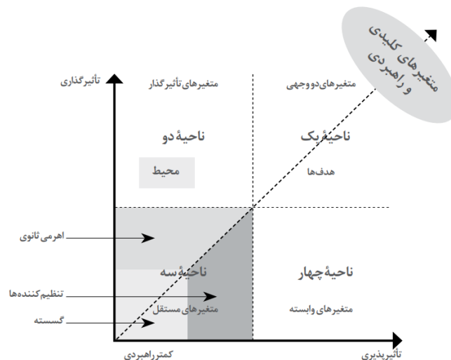
شکل ۱. نقشه و تفسیر موقعیت‌های چهارگانه محور مختصات میکم (رهسپار و همکاران، ۱۳۹۸)
