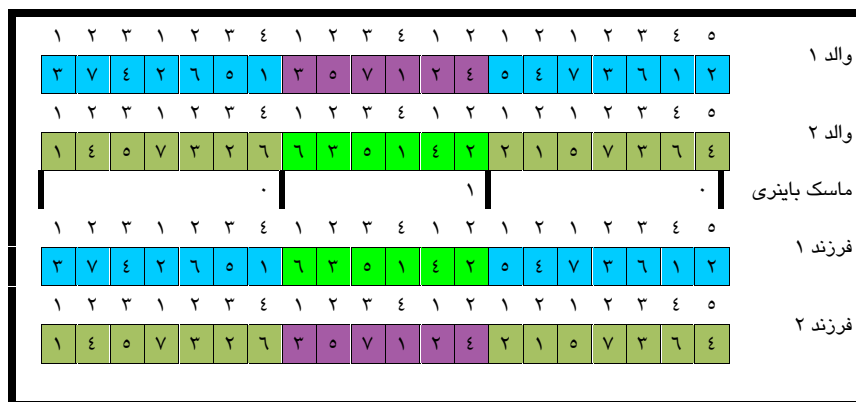
شکل ۶ اپراتور تقاطع
