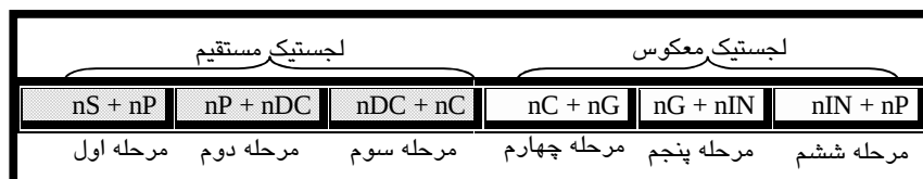
شکل ۵ نمایش کروموزوم
